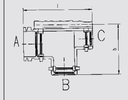
Forme D / Form D
